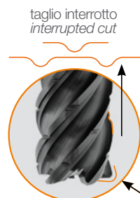
raggio torico toric radius
