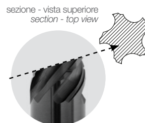
gola raggiata rounded flute
